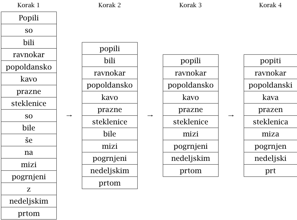
SLIKA 3. Potek delovanja cevovoda predobdelave besedil
