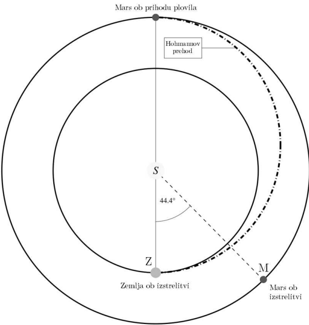
SLIKA 3. Hohmannov prehod plovila z Zemlje na Mars
