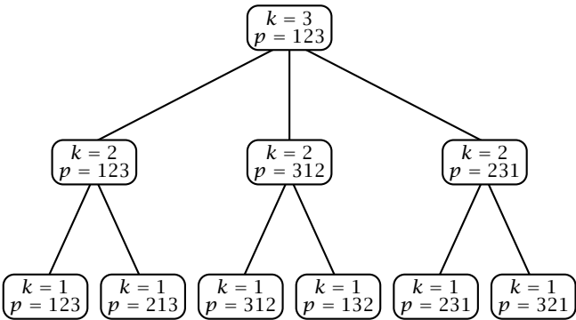
SLIKA 2. Delovanje algoritma Heap za n = 3 .
