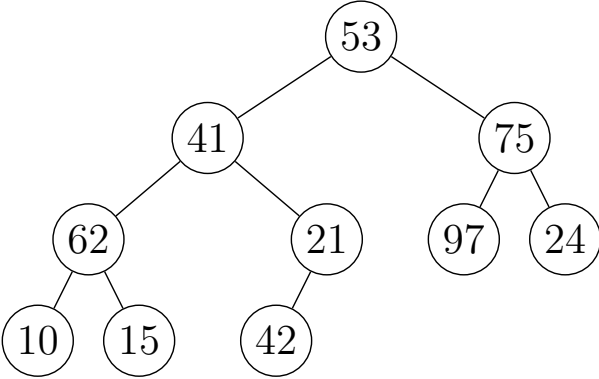
SLIKA 5. Polje, ki ne predstavlja nujno kopice, in pripadajoče dvojiško drevo.
