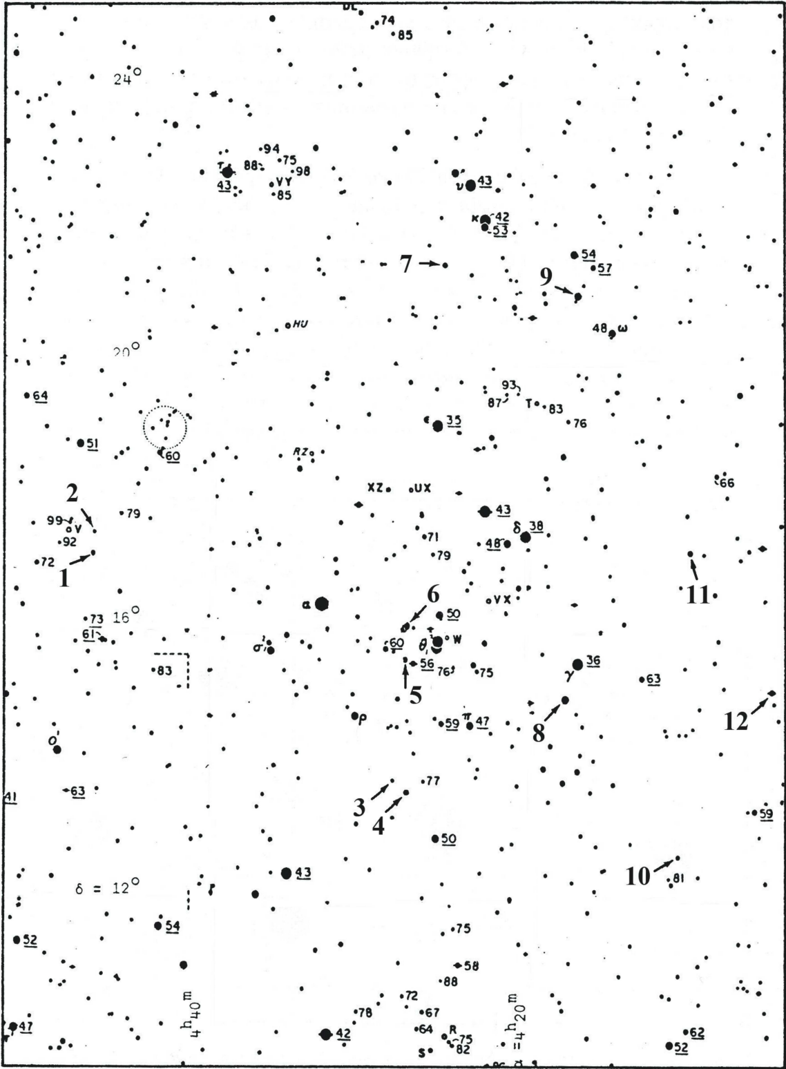
SLIKA 3. Zvezdna karta dela neba v območju Hijad.
