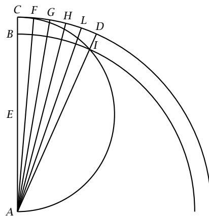
Risba iz Galileijevega Dialoga kaže padanje kamna na vrteči se Zemlji v ravnini vzporednika. Lok CD ustreza gibanju vrha stolpa, lok BI gibanju njegovega vznožja, lok CI s središčem v E na polovici polmera CA pa tirnici kamna. Kot CEI v vrhu E je dvakrat večji kot kot CAD ob vrhu A in polmer CD je dvakrat večji kot polmer CE . Zato je pot vrha stolpa enaka poti kamna.
