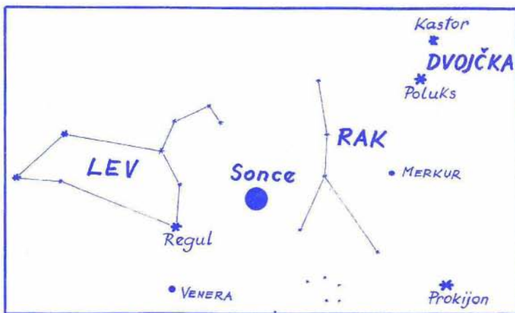
Slika 2. Ob popolnem mrku bomo v jasnem vremenu visoko na nebu okoli od Lune zatemnjene Sonca lahko opazovali svetle zvezde Prokijon, Regul, Kastor in Poluks, od planetov pa Venero in Merkur.
